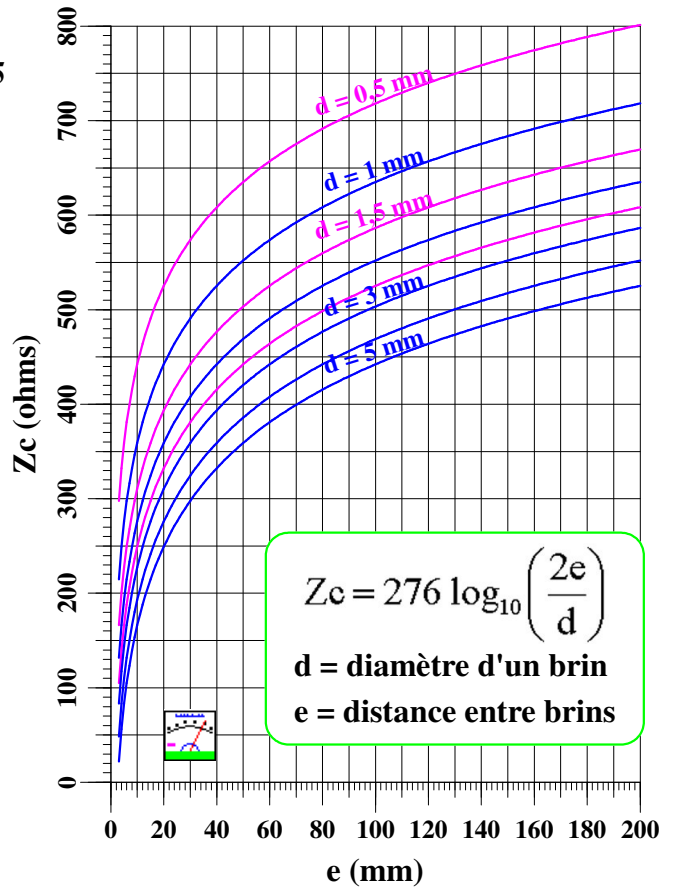
Impédance caractéristique d'une ligne bifilaire
